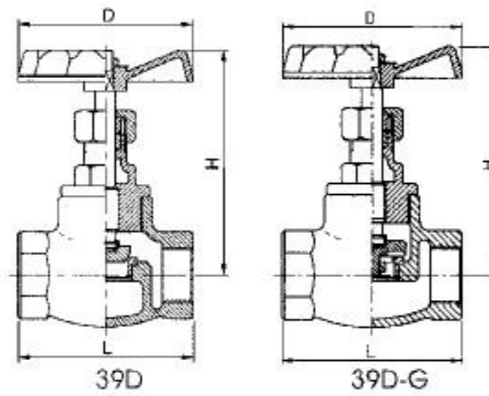
詳細尺寸 Dimension 單位 Unit : 公釐 mm
