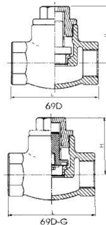
詳細尺寸 Dimension 單位 Unit : 公釐 mm
